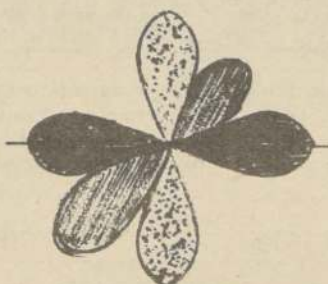
Orbitales "p"
