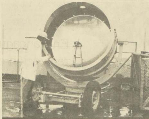
Horno solar, con espejos parabólicos que están a cargo del ayudante técnico Rafael Bolocco, en la Universidad Santa María.
