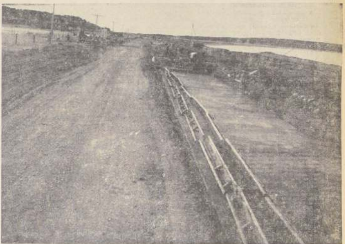
Camino que une Punta Arenas con Chabunco y Río Pescado, cuyos trabajos de pavimentación se encuentran en sus fases finales. Esta es una de las numerosas obras que ha inspeccionado el Ministro de Obras Públicas y Transportes, Sergio Ossa Pretot, quien se encuentra en esa zona. El programa de construcción de obras para la provincia de Magallanes durante el presente año significa una inversión superior a los 2 millones 500 mil escudos.
