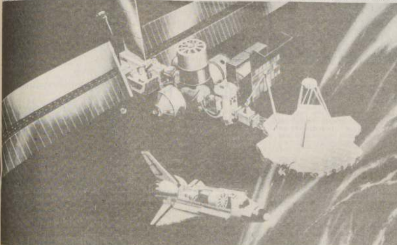
Este dibujo muestra la propuesta construcción por los astronautas del trasbordador en órbita terrestre, de una antena llamada gran reflector emplazable.
