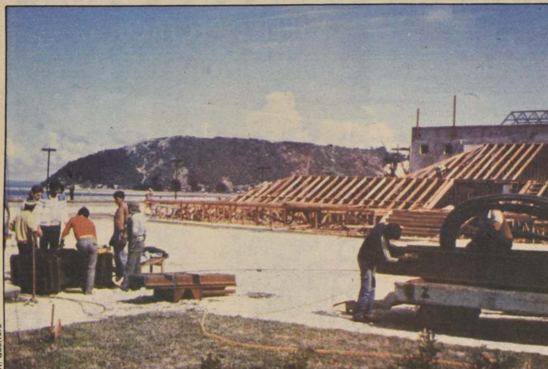
Altar papal: En alerce y sobre 40 contenedores se está ejecutando el altar desde donde el Papa Juan Pablo II oficiará su Eucaristía en la ciudad de Puerto Montt, luego de un recorrido de 40 minutos que efectuará por la bahía, a bordo del buque Cirujano Videla. Lo acompañarán cinco mil embarcaciones de pescadores.
