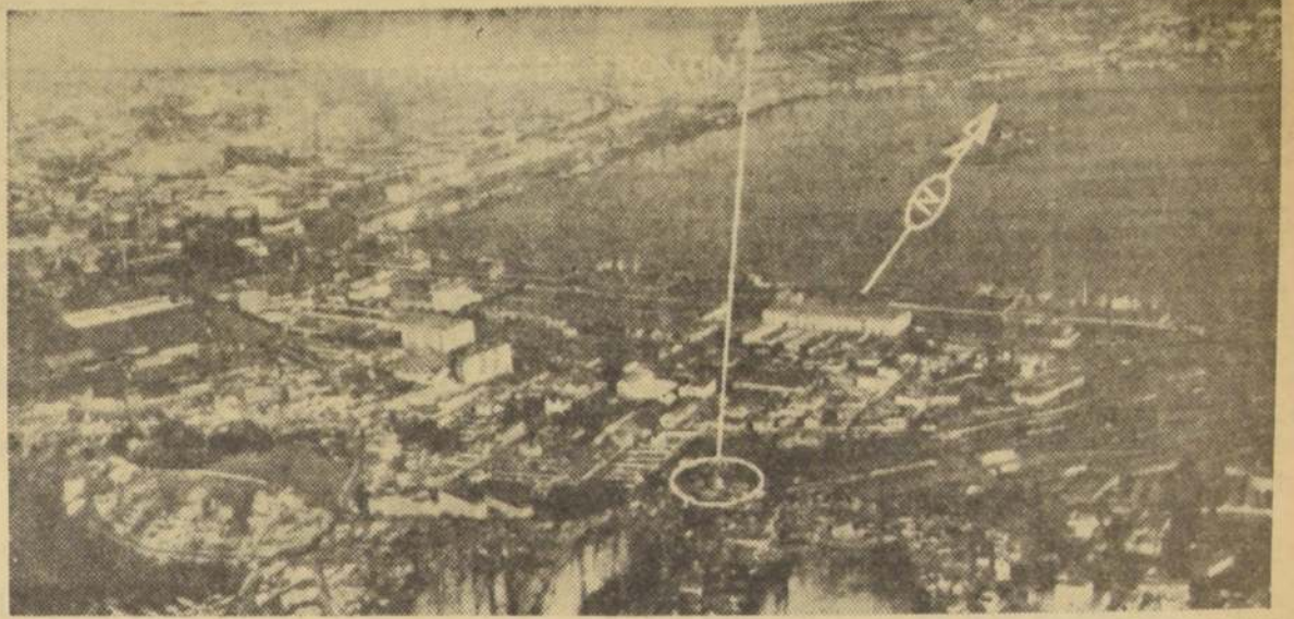
RED DE COMUNICACIONES EN BRASIL. — Una de las estaciones terminales del sistema de telecomunicaciones en la costa de Río de Janeiro. Además de Brasilia y Río de Janeiro, hay en funcionamiento otras estaciones terminales en Be-
