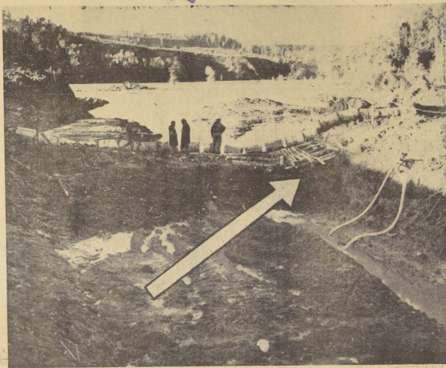
TACO-COMPUERTA.— El grabado muestra el "taco-compuerta" que hoy, a las 7 de la mañana, dará paso controlado a las aguas contenidas en el Lago Riñihue. Esta obra de más o menos 2 metros de altura, será volada a las 7 horas, y a través del hueco que deje comenzará la afluencia de las aguas en dirección a Valdivia, a través del canal construido con máquinas y hombres de la ENDESA, la CORFO y de la Dirección de Vialidad.
