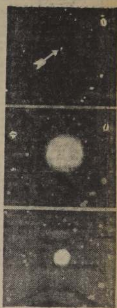
LA FLECHA de arriba indica cómo lucía la Pictoris en 1925. Al centro: aparece la "nova" en donde estaba la estrella Pictoris. Abajo: se nota que la estrella se fragmenta.
