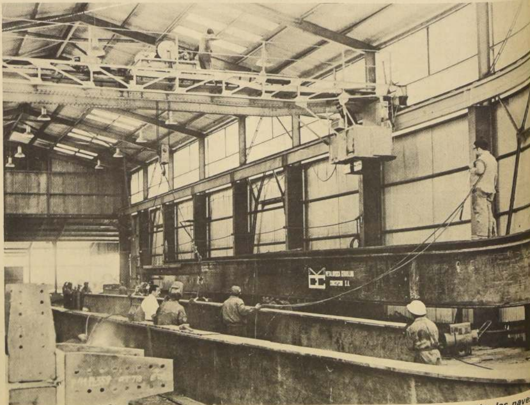
Las vigas del Paso Inferior Santa Lucía, en una etapa de su construcción, en una de las naves industriales de METALURGICA CERRILLOS CONCEPCION S. A., en la comuna de Talcahuano.
