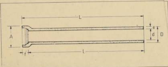
TUBOS CON ENCHUFE DE CAMPANA
