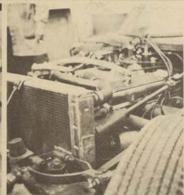
EL MOTOR Z-28 EN TODA SU EXTENSION. El ancho radiador, la barra de la dirección, el recolector de el carburador completo, junto con el sistema de amortiguación y un neumático standard, este "close up".
