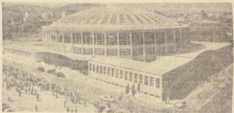
EL PALACIO DE LOS DEPORTES DE BOLONIA, una de las obras de mayor interés arquitectónico en su especie, construido en el año 1956. Arquitecto Rocatelli y Valle, Ingeniero Francisco Allegria.
