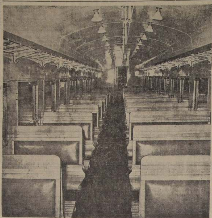
Detalle del interior del nuevo coche de acero para los Ferrocarriles del Estado, construido integralmente en Chile, en los talleres de Socometal. La única diferencia con los coches de lujo en servicio actual, está en los asientos. La seguridad y construcción metálica son idénticas a los coches de primera
