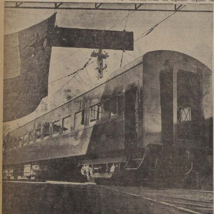
Vista exterior del nuevo coche de pasajeros para tercera clase, totalmente de acero, construido en los talleres de Socometal. El vagón posee aislamiento térmico de lana de vidrio y todas las características de seguridad de los coches de lujo
