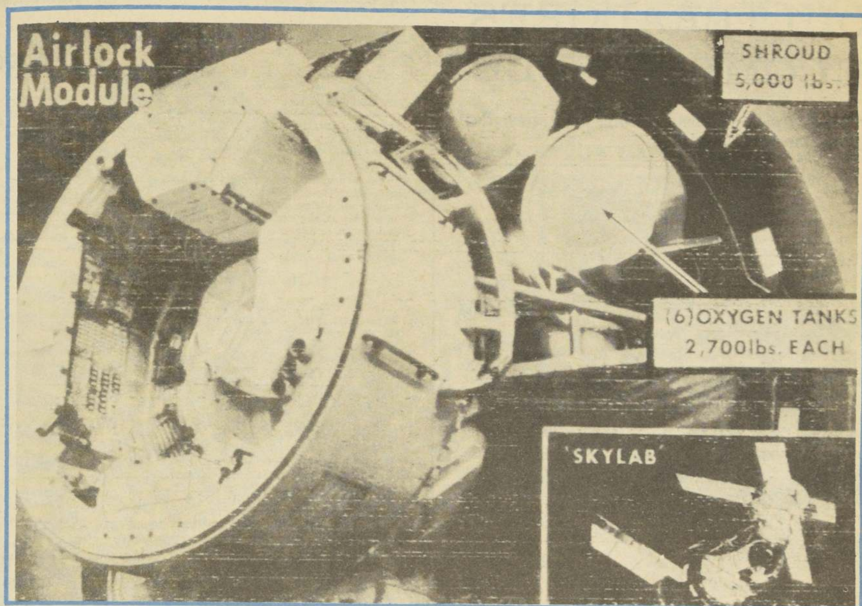
↑ LA FOTOGRAFIA muestra el módulo del Skylab que sobrevivirá al roce atmosférico que, debido al calor generado, desintegrará el laboratorio espacial. Este pesa 2.700 kilos y sería uno de los 500 trozos más pesados que caerían sobre la tierra.
