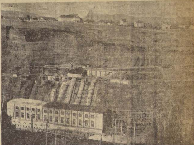
CONSTRUIDA POR LA "ENDESA" — Esta Planta hidroeléctrica de "El Pilmaiquén", es una de las obras más perfectas, en su género, que hace diez años construye la "ENDESA", en Sud América.
