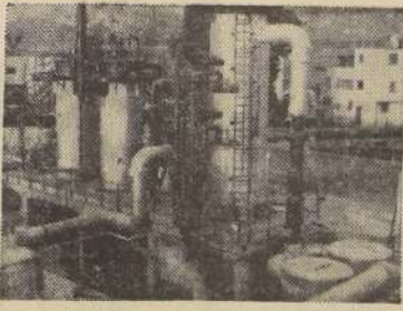
Vista de una planta de Acido Sulfúrico catalítico instalada por CHEMIEBAU en DARMSTADT (Alemania Occidental)
