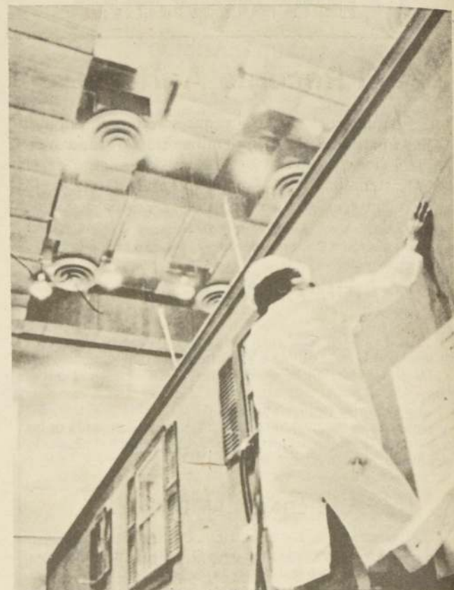
En el Centro para tecnología de la construcción en Gaithersburg los ingenieros inspeccionan una casa móvil colocada dentro de una gran cámara ambiental para poner a prueba su respuesta térmica.
