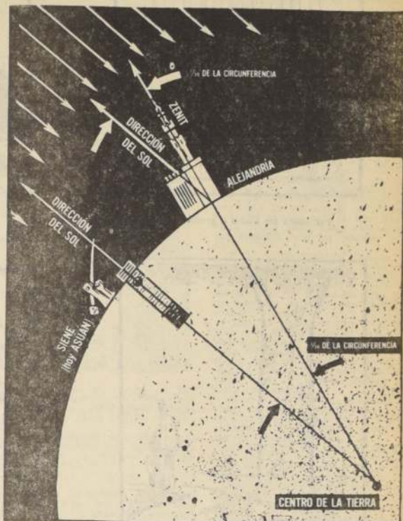
Diagrama que explica la teoría de Eratóstenes sobre la redondez de la Tierra.
