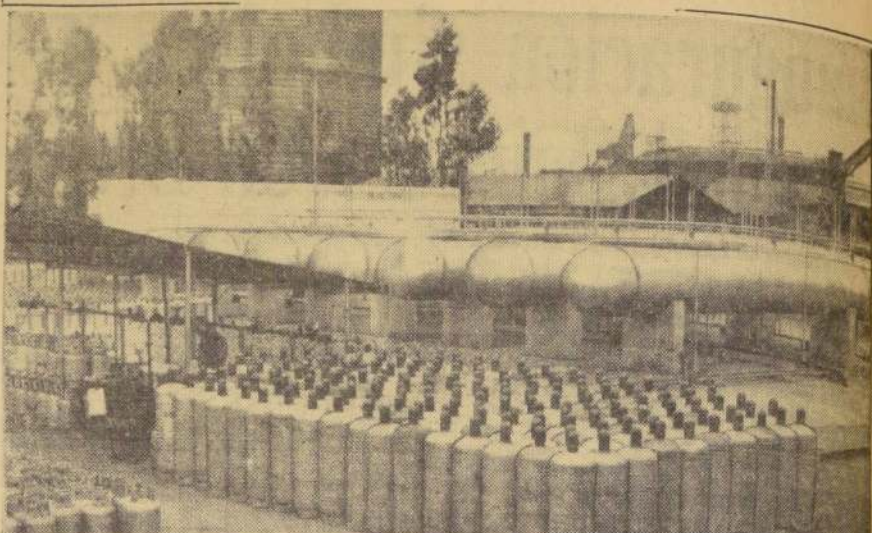
Planta de llenado y almacenamiento de gas licuado de la Compañía de Gas de Santiago, la que dispone de una capacidad de llenado de 1.000 toneladas mensuales. Esta es la primera en su género establecida en la capital, y en fecha cercana será ampliada al trasladarse a los terrenos que la Compañía de Gas posee en Maipo, donde está en construcción una moderna planta.
