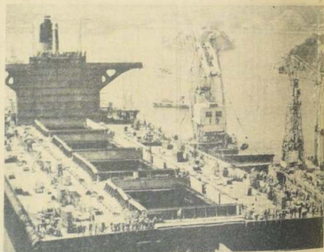
Enormes barcos tanque construyen los astilleros japoneses. En el grabado, el trabajo en las instalaciones constructoras de buques de la isla Innoshima, de la Prefectura de Hiroshima, en el Mar Interior de Seto
