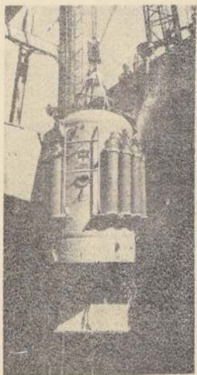
Esta cámara neumática del "Cachelot" evita la tediosa y arriesgada descompresión de los buzos, cuando suben desde grandes profundidades.
