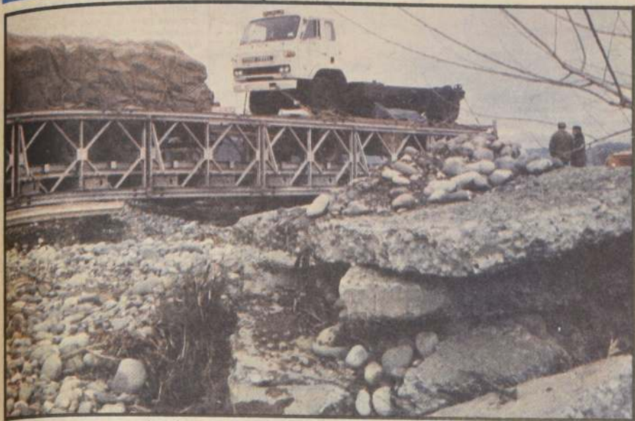
Un puente metálico de emergencia instalado por Vialidad permitió superar la situación derivada de la destrucción de ambas calzadas de la Carretera Longitudinal, que fueron arrasadas por las aguas del estero Santa Blanca, a la altura de Codegua. (Foto Marcelo Agost).
