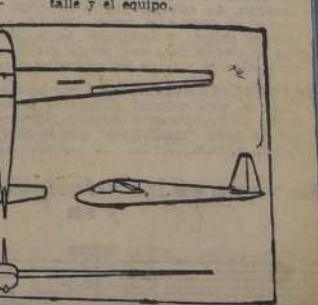
DISPOSICION general del "Crabpot I", diseño original de Hugh Kendall, que ganó el concurso de diseño de la Asociación Británica de vuelos sin motor, en 1947. La versión modificada que se fabrica ahora, llamada "Miles M. 76", tiene alas, estabilizador en "V" y alerones plásticos.
