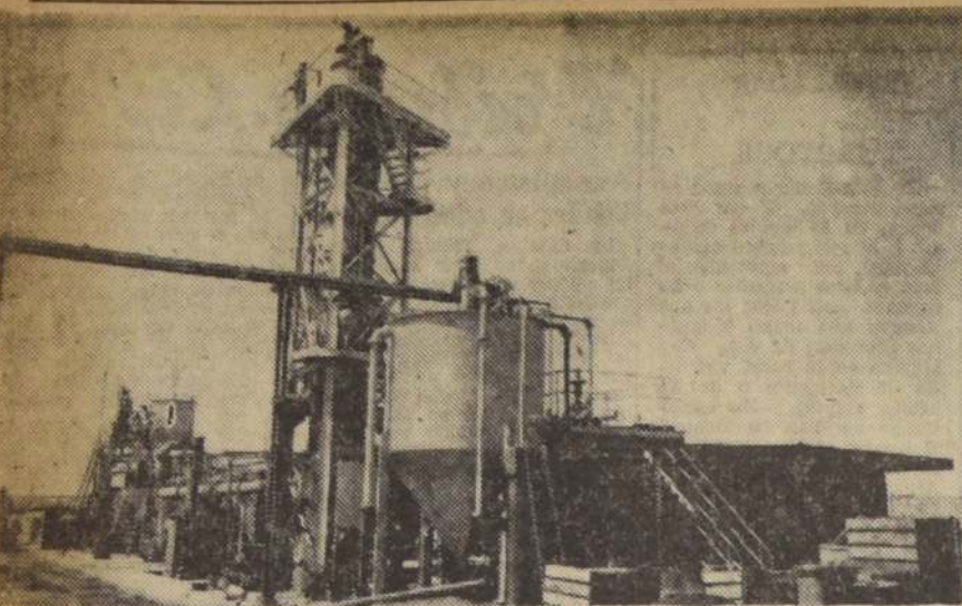
Moderna planta de yodo de Coya Sur, la que puede ser aprovechada para otros materiales y que, con su uso actual, produce ya 6.500 kilos diarios.
