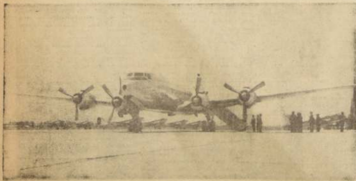
POCO DESPUES DEL MEDIODIA de ayer llegó a la losa de Los Cerrillos, para después trasladarse a la del Grupo de Aviación Nº 19 de la FACH, el transporte DC-59 que adquirió la Fuerza Aérea en un plan de compra de aviones de transporte. La máquina está destinada a trasladar carga de las Fuerzas Armadas a través del territorio nacional. En el Grupo 19 fue recibida por el Comandante en Jefe de la FACH, general del aire Maximo Errázuriz y otras altas autoridades de la institución, EN EL GRABADO, el nuevo transporte adquirido por la FACH.
