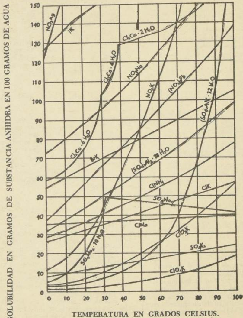
Influencia de la temperatura sobre la solubilidad de algunas sales en agua.
