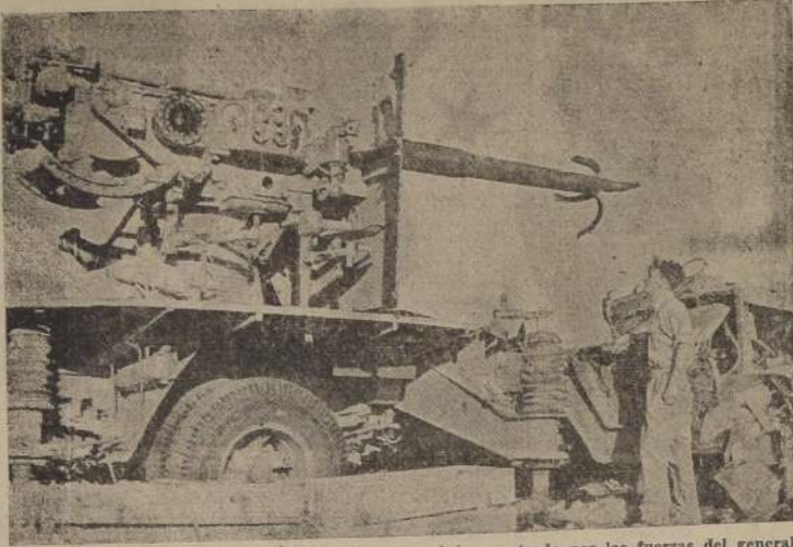
Un cañón antitanque alemán de 88 mm. tal como fue encontrado por las fuerzas del general Anderson en el curso de una reciente acción librada en África del Norte. Los alemanes, cuando se ven obligados a replegarse rápidamente, suelen destruir estas poderosas piezas de artillería, de gran eficacia pero de lenta movilidad.
