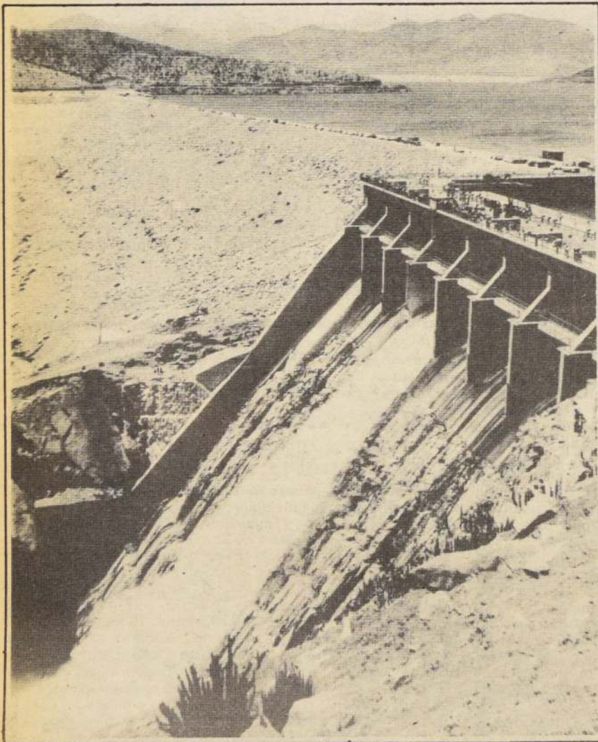
El embalse La Paloma, otra realización que permite asegurar la agricultura en el Valle del Limarí y alimento para una enorme población en la zona central.
