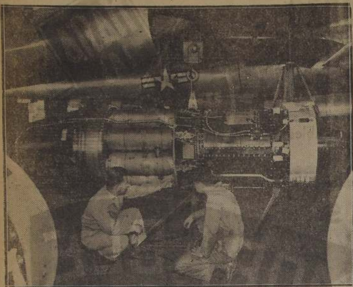
Técnicos de la Boeing en el momento de examinar una máquina de retropropulsión, antes de montarla en un "Stratojet" XE-47, el bombardero más veloz del mundo. Seis J-47, máquinas de retropropulsión de la General Electric, irán a reemplazar a las menos poderosas J-35. Estas nuevas máquinas se producen ahora para la Fuerza Aérea de los Estados Unidos y se utilizan en modelos experimentales. Ahora se ha construido un nuevo túnel de viento hipersónico en Estados Unidos que permitirá realizar experimentos para aumentar aún más la velocidad de estos aviones.
