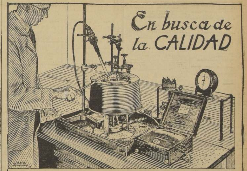
La prueba "Ramsbottom" sirve para determinar la cantidad y naturaleza del residuo carbonoso que producen los aceites durante su empleo.
