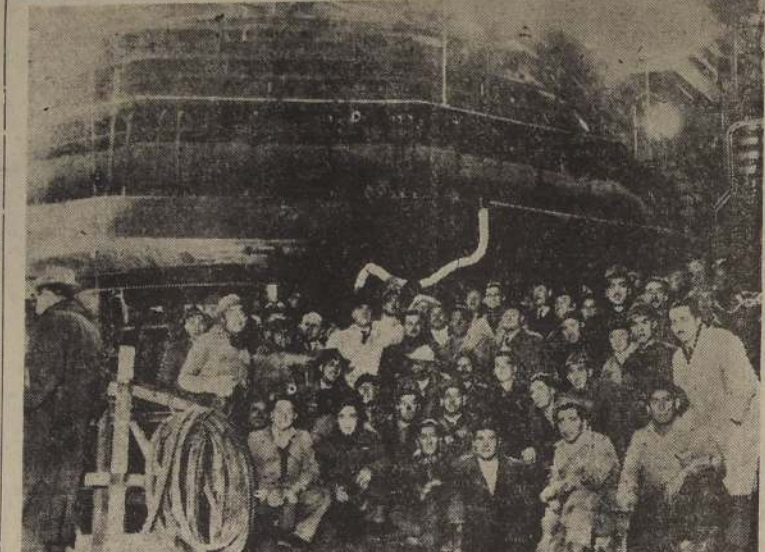
HUACHIPATO PRODUCE HIERRO FUNDIDO.— Asistentes a la salida de la primera "colada" de hierro fundido del Alto Horno de Huachipato. Aparecen los señores Arturo Matte, Roberto Vergara, Eduardo Figueroa y otros jefes e ingenieros de la CAP, acompañados de obreros de la planta y periodistas penquisistas, incluyéndose nuestro correspondiente.
