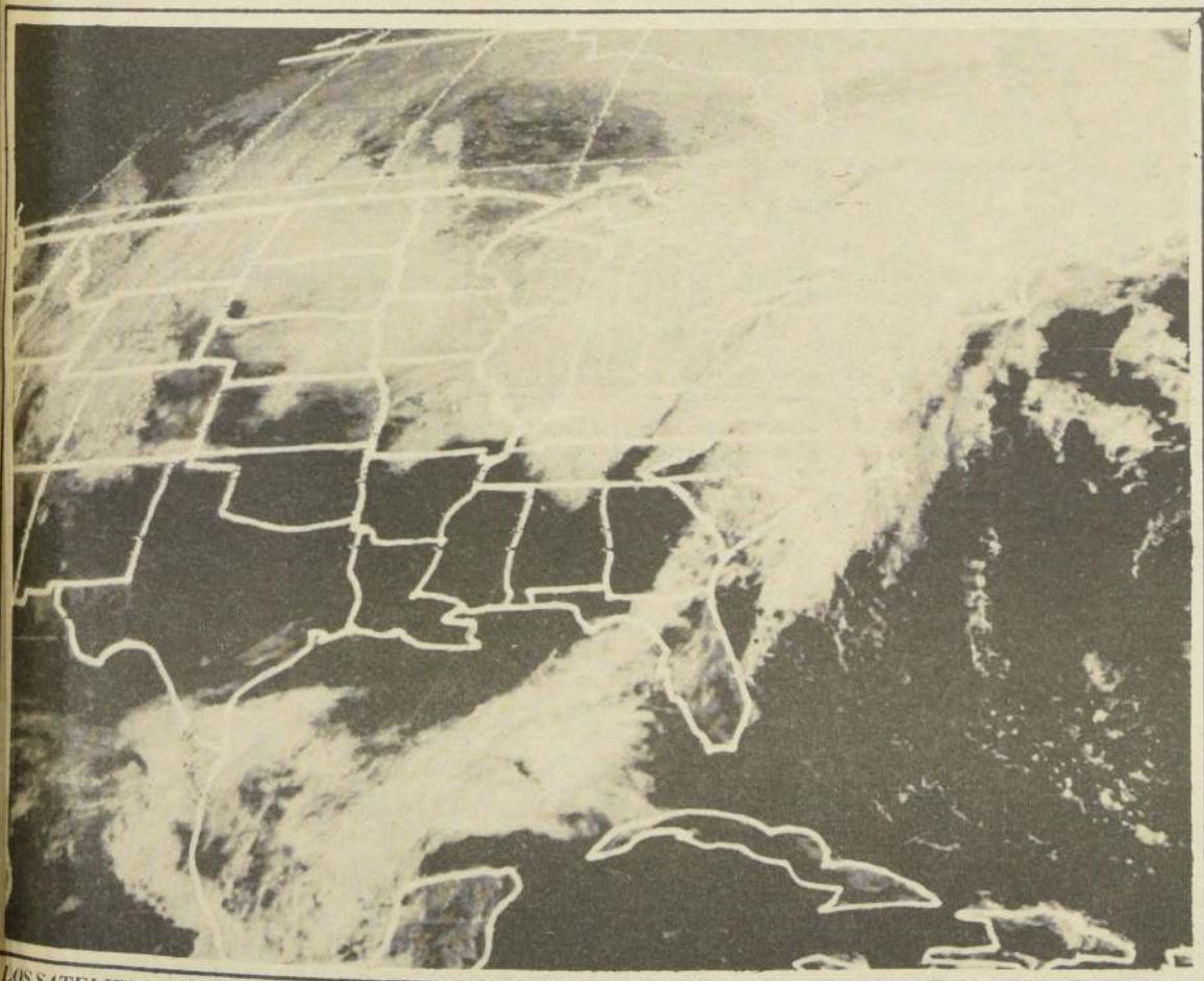
LOS SATELITES ARTIFICIALES proporcionan valiosos datos sobre las características de nuestro planeta. La NASA arrendará servicios similares a organismos interesados.
