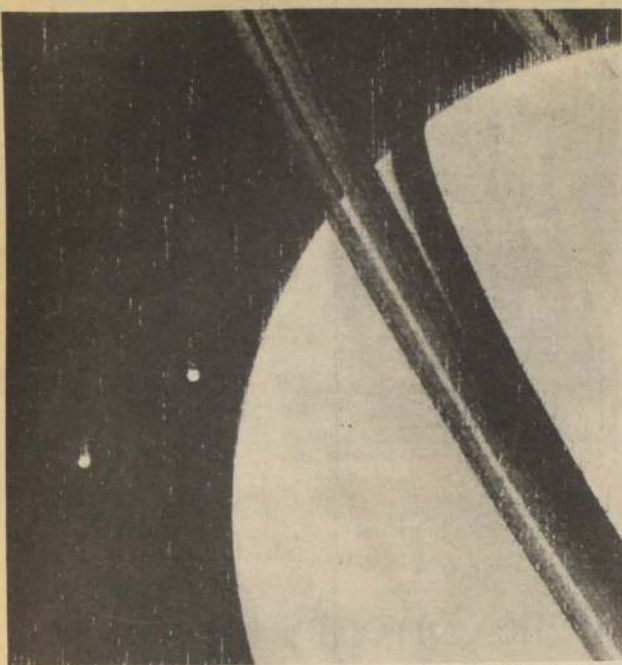
Desde una distancia impresionante de 3 millones de kilómetros, la nave Voyager 1 de EE.UU. se encuentra enviando fotos del planeta Saturno, las que tienen intrigados a los científicos por la cantidad de situaciones nuevas que han podido descubrir respecto a las lunas que lo rodean y los anillos que contiene (Radiofoto UPI).
