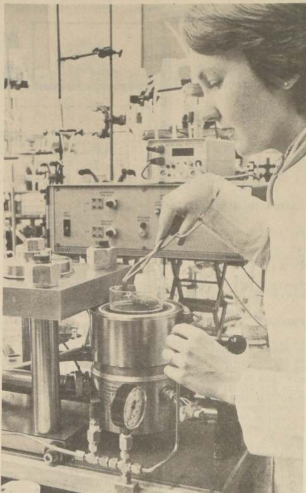
La asistente pone una probeta en el recipiente de presión que se puede tapar herméticamente con el carro correspondiente que está a la izquierda. Además de las investigaciones de productos alimenticios, el nuevo procedimiento está concebido también para la medicina laboral, legal o veterinaria.
