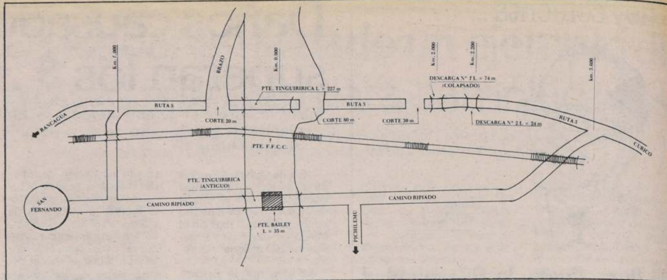
El gráfico muestra exactamente la situación que afecta al puente Tinguiririca, que sufrió tres cortes de 20, 80 y 30 metros y, en la parte inferior, la ruta alternativa que debe ocuparse en la actualidad, tras la instalación del puente tipo Bailey ubicado sobre los soportes del antiguo viaducto, uniéndose así Curicó con San Fernando.
