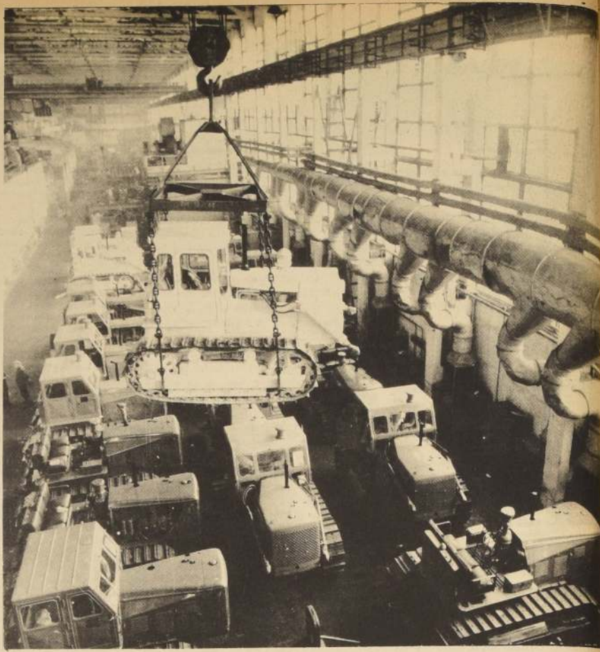
Tractores "T-130" en el taller de equipamiento de la fábrica de Cheliabinsk.
