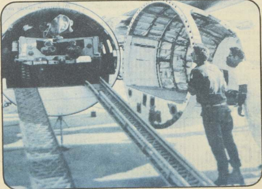
Una demostración de su versatilidad efectuó ayer en Peldehue el avión civil y militar israelí "ARAVA". Este aparato, construido por la Industria Aeronáutica de Israel, puede transportar un jeep armado, 18 paracaidistas, 20 pasajeros e incluso transformarse en avión de ejecutivos.
