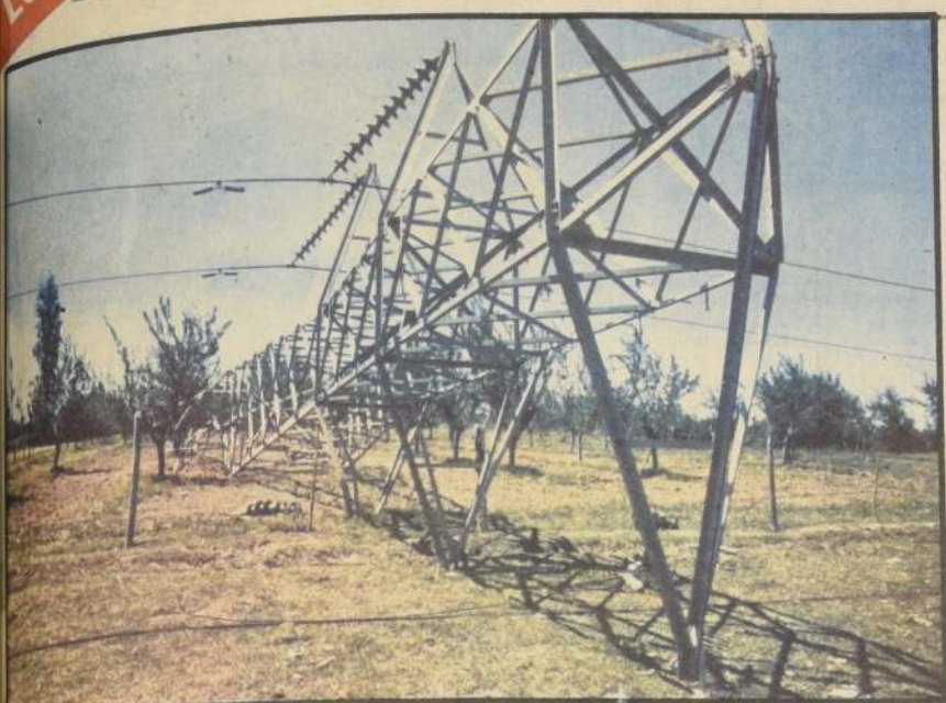
Estado en que quedaron las torres de alta tensión saboteadas por los extremistas. La foto da una idea de la potencia del explosivo utilizado, por quienes esgrimen la violencia como recurso político.
