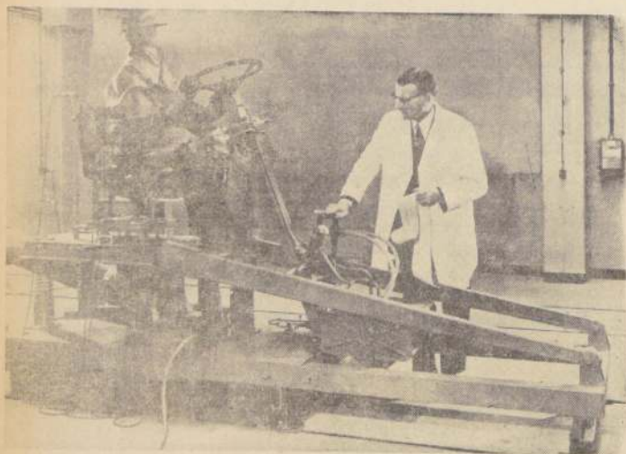
El muñeco de plástico que muestra la fotografía, se encuentra lleno de delicados instrumentos electrónicos con los que se miden todos los esfuerzos a que se encuentra sometido un conductor humano. El inventor, un ingeniero alemán, ha logrado mediante este dispositivo obtener un asiento perfeccionado para conductores que anula todos los efectos de la vibración, incluso en camiones y tractores.
