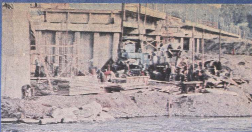
Pilotes de reforzamiento: última etapa de las obras de reconstrucción del puente que une San Antonio con Rocas de Santo Domingo.
