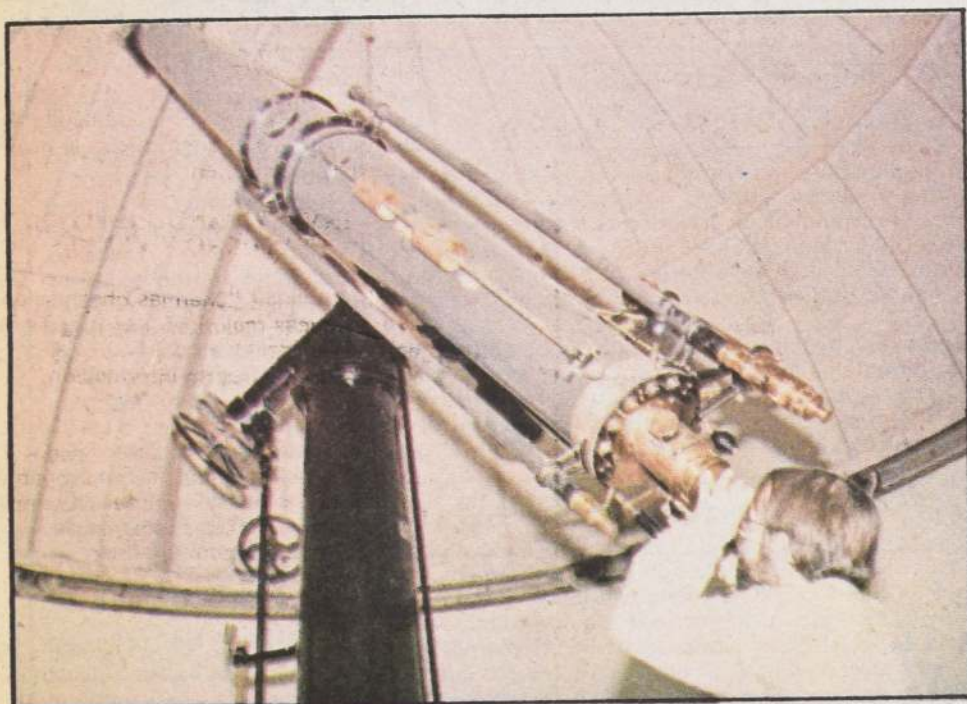
El doctor en astrofísica, José Maza, observa el cielo a través del antiguo telescopio adquirido por el astrónomo alemán Federico Ristenpart, alrededor de 1910, y que constituye una verdadera reliquia del Observatorio Astronómico Nacional.
