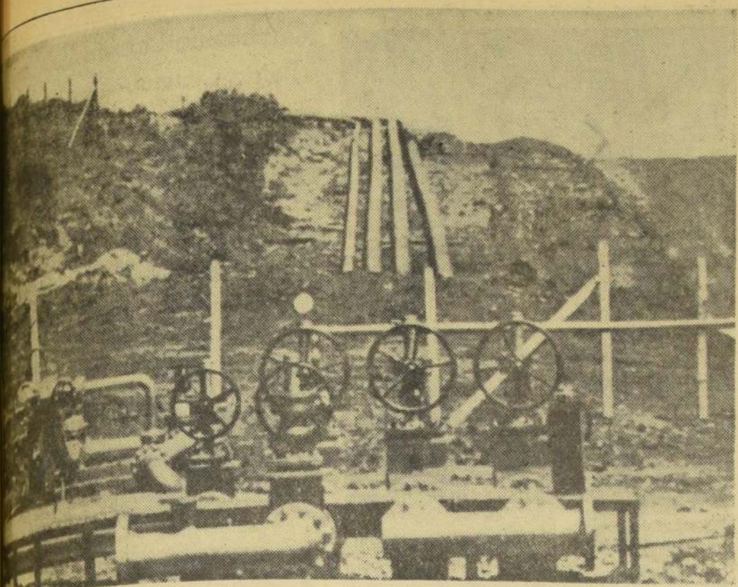
GENERAL DE LA OBRA.— El oleoducto para transporte de combustible se extiende desde Concón hasta Maipú. En el primer tramo se aprecia la instalación en Concón, donde se encuentra ubicado el equipo de bombeo que impulsa el producto hasta el otro extremo de la línea, a ciento diecinueve kilómetros de distancia.
