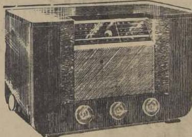
Q-109. — 9 tubos; corriente alterna; onda corta y larga; 5 bandas espaciadas; control de tono; Ojo Mágico; conexión para pick-up; gabinete enchapado.
