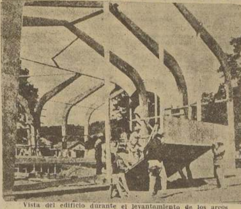
Vista del edificio durante el levantamiento de los arcos temporales hasta que las planchas de madera laminada pudieran ser colocadas en su lugar.
