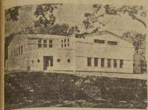
Un curioso tipo de construcción, en cuya estructura se utilizaron arcos elásticos de madera laminada, colocados en secciones listas para emplearse.
