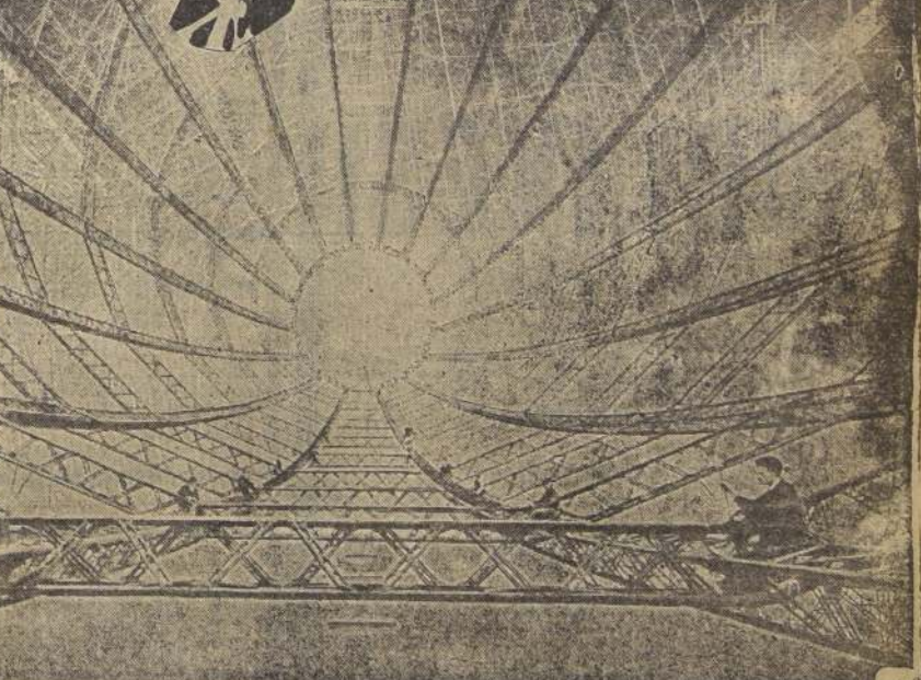
Una vista tomada durante el proceso de la construcción de la aeronave. Toda la armadura interior, del tipo rígido, es de duraluminio y en ella van los balones de gas.
