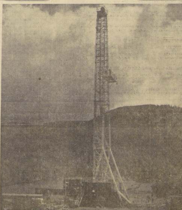
Esta elevada torre, con técnicos chilenos y modernos equipos, determinará la existencia de petróleo en Lebu. Se trata del primer pozo, cuya perforación fue iniciada ayer por la ENAP, tal como lo hará próximamente en las provincias de Llanquihue y Osorno. Los resultados —satisfactorios o no— se sabrán dentro de algún tiempo más, una vez que la perforación haya alcanzado los 3.300 metros de profundidad. En Arauco existe verdadera expectativa por la posibilidad de que se abra una nueva fuente de producción y trabajo en la zona.
