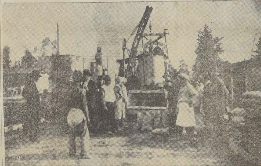
LA BETONERA "RAMSONES", QUE HACE LA MEZCLA DEL CONCRETO Y LO DEPOSITA EN LA CALZADA, TODO AUTOMÁTICAMENTE Y CON UN RENDIMIENTO DE VARIAS CUADRAS POR DÍA.
