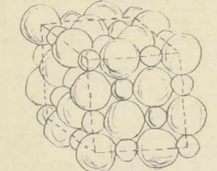
Disposiciones de los iones en el cloruro de sodio cristalino
