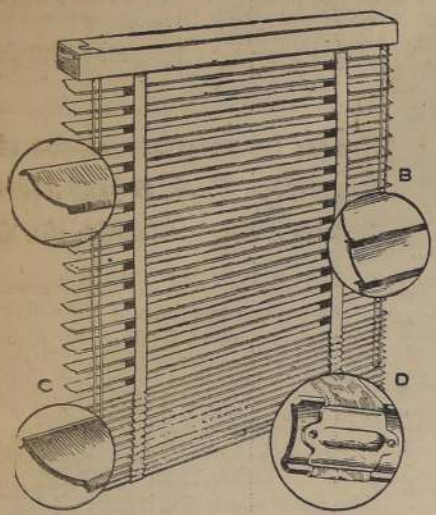
Los círculos A, B, C y D encierran detalles de las características más interesantes de una persiana de aluminio
