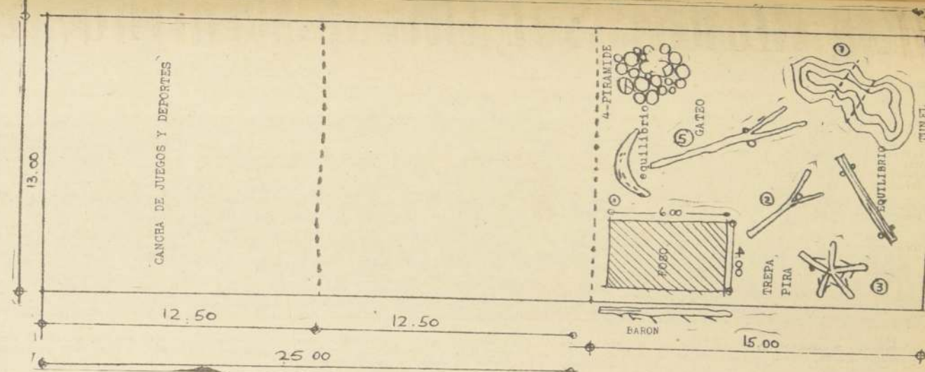
He aquí una plaza de juegos y de deportes, apropiada para cincuenta niños. Puede observarse en la parte destinada a los juegos, la distribución de los distintos equipos, en forma armónica y un foso de seis metros, como también un instrumento de equilibrio, uno de trepar, un túnel, etc. Este sistema de plaza de juegos y deportes, es una contribución valiosa, para despertar el interés de los niños, por los deportes.
