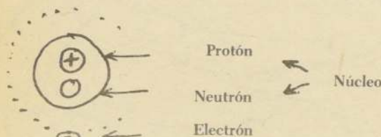
Partes de un átomo
