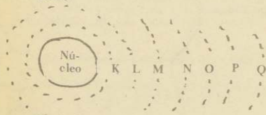
Partes de un átomo
