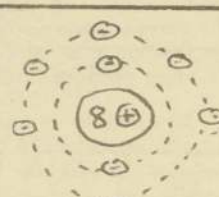
Átomo de O
