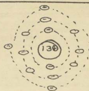
Átomo de Al
