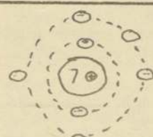
Átomo de N
