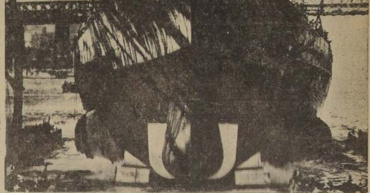
El superacorazado norteamericano "North Carolina", de 35.000 toneladas, en los momentos en que es lanzado al agua, en marzo último. Los norteamericanos sostienen que es el barco de guerra más poderoso a flote.
