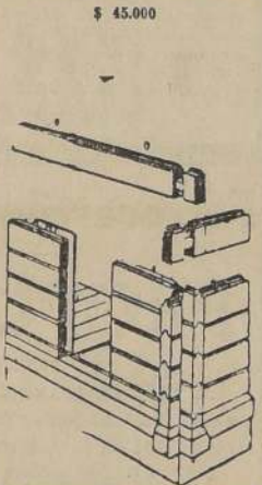
Este esquema indica el montaje de la construcción en madera llamada vulgarmente maciza, en tabloncitos de 10 x 20 cms.
