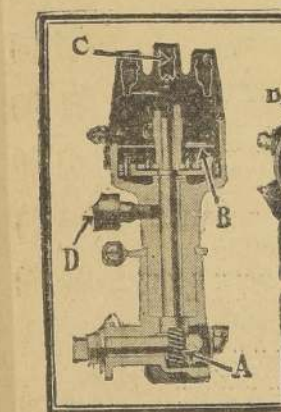
A) Engranaje del distribuidor. — B) Eje de dirección. — C) Mecanismo de distribución. — D) Taza del distribuidor que conduce a las bujías para lubricar el eje de distribución.
